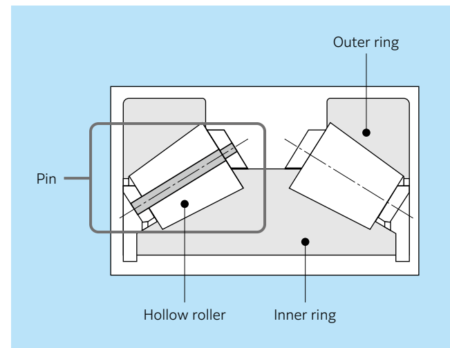
Fig. 2 Pin type cage
