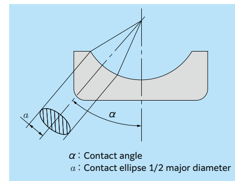
Fig. 3.14 Contact ellipse
