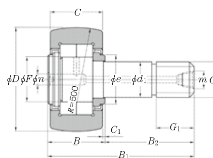
NUKR type ( D \geq 100 mm)
